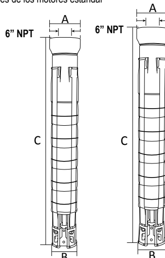
Acoplamiento NEMA 6" Fig. 1
