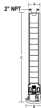
Acoplamiento NEMA 6"
