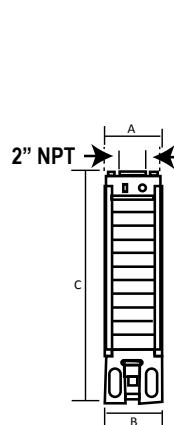
Acoplamiento NEMA 4"
