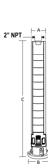
Acoplamiento NEMA 4"
